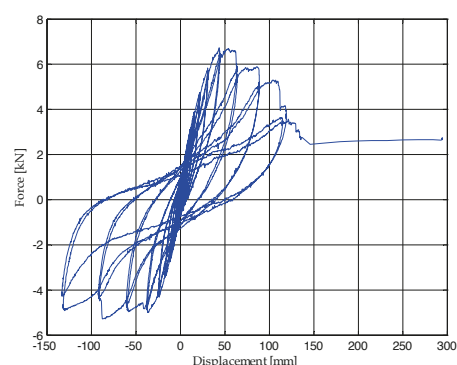
Prove fuori piano - Cicli di isteresi
